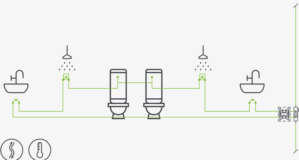
Ringinstallation mit Strömungsteiler
