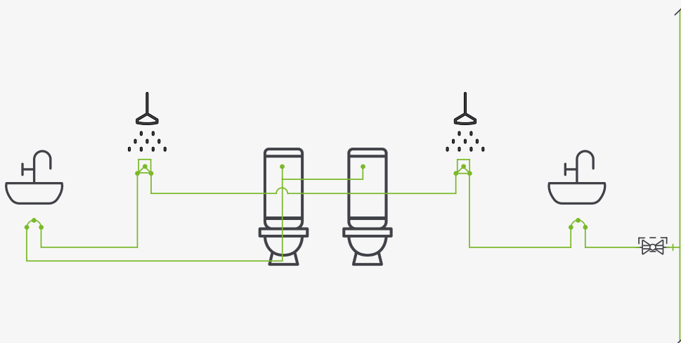
Konventionelle Reiheninstallation
