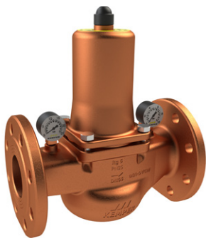
Flanschen-Druckminderer, Figur 711 00
