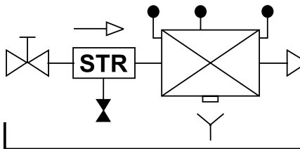
Sicherungseinrichtung Systemtrenner BA
