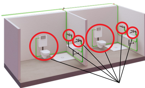
Mehrere Spülpunkte pro Nasszelle
