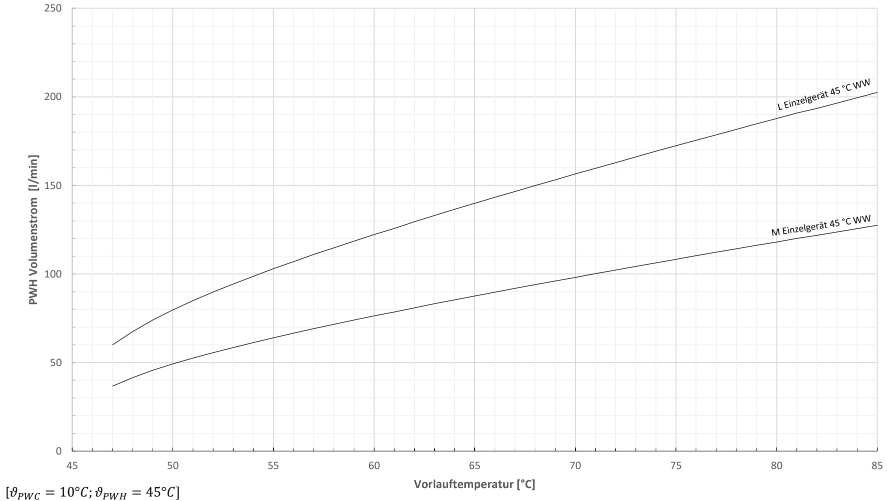
Leistungsdiagramm Einzelgeräte PWH 45 °C
