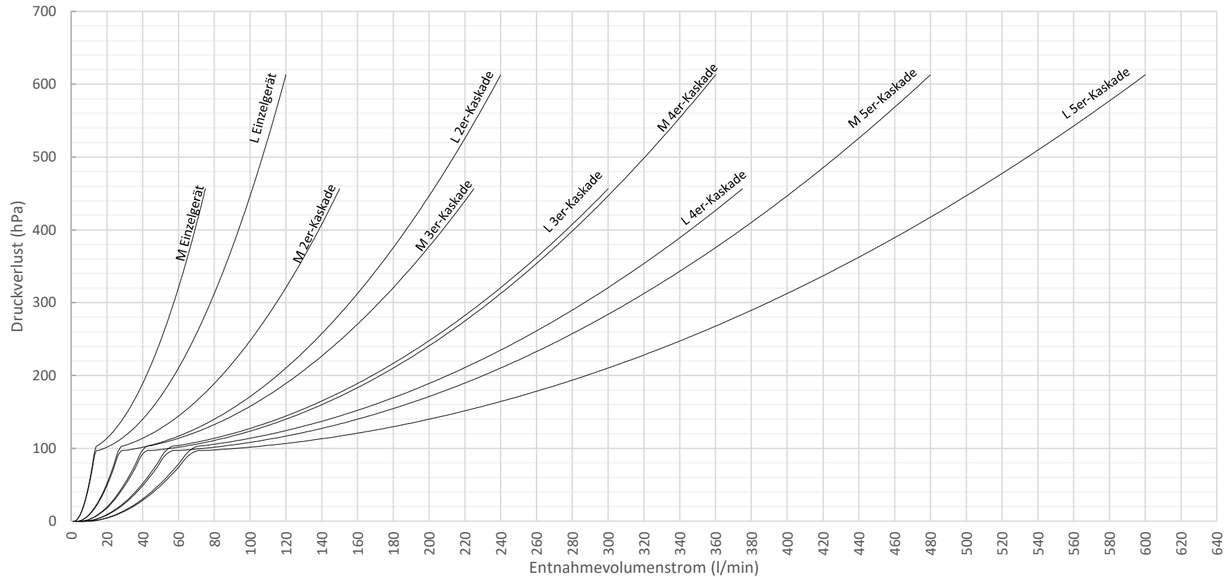
Druckverluste Trinkwasserseite (sekundär)
