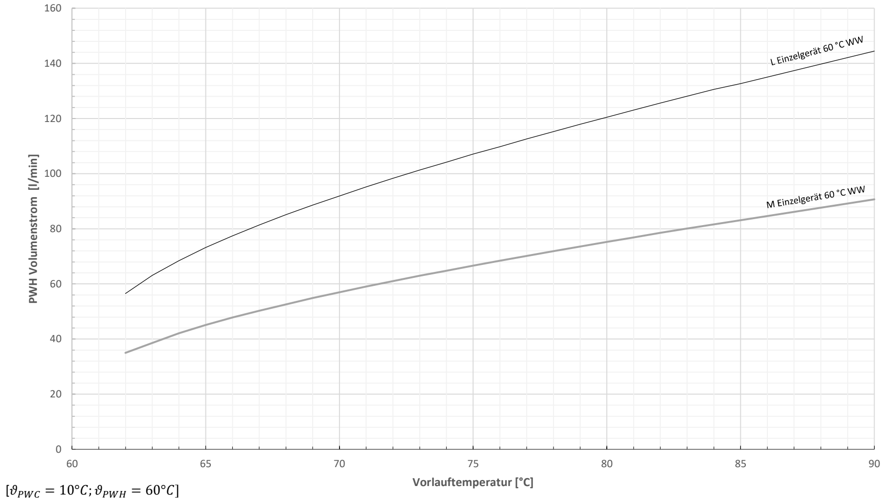
Leistungsdiagramm Einzelgeräte PWH 60 °C
