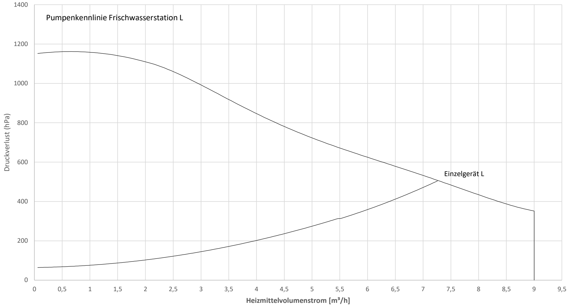
Pumpenkennlinie und primärer Druckverlust L
