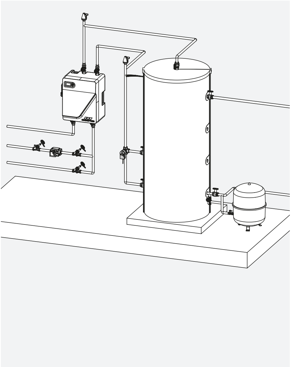
Abbildung 2 - Schematische Darstellung.
