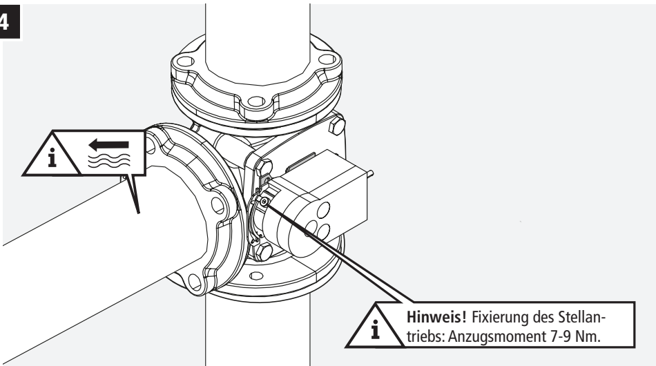
Abbildung 14 – Fixierung des Stellantriebs: Anzugsmoment 7-9 Nm.
