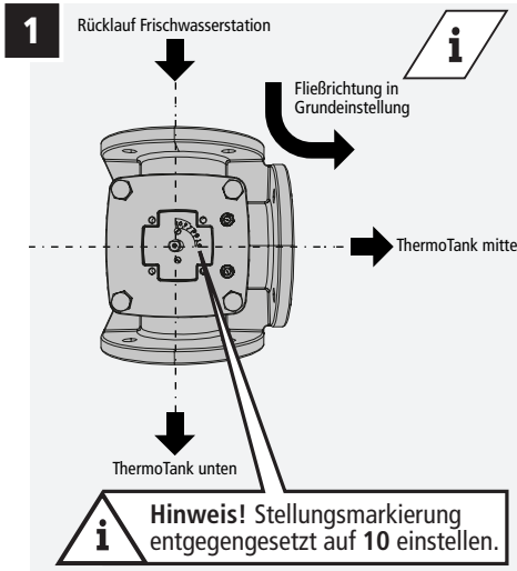
Abbildung 15 - Stellungsmarkierung.
