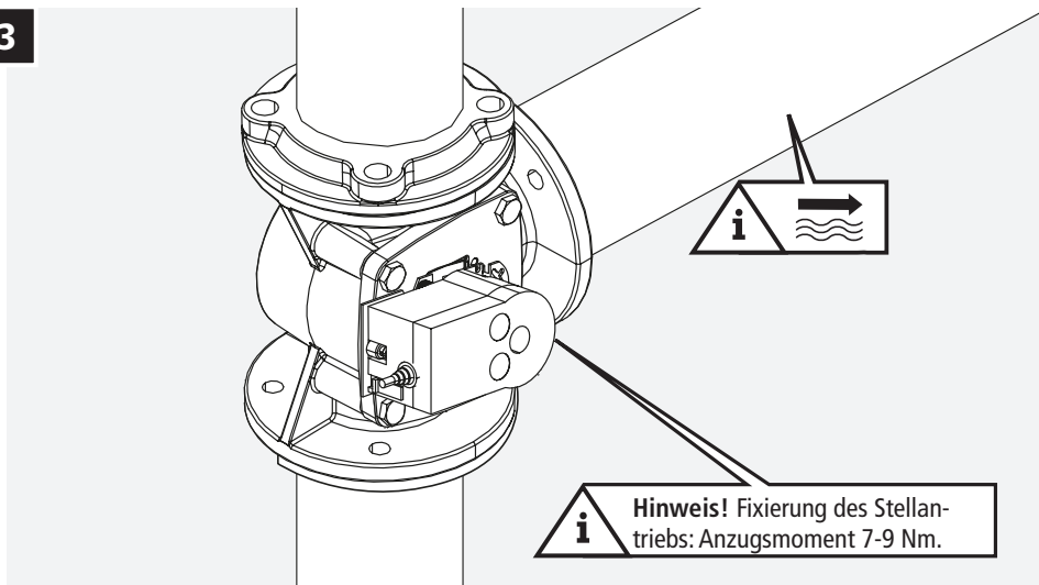
Abbildung 18 – Fixierung des Stellantriebs: Anzugsmoment 7-9 Nm.
