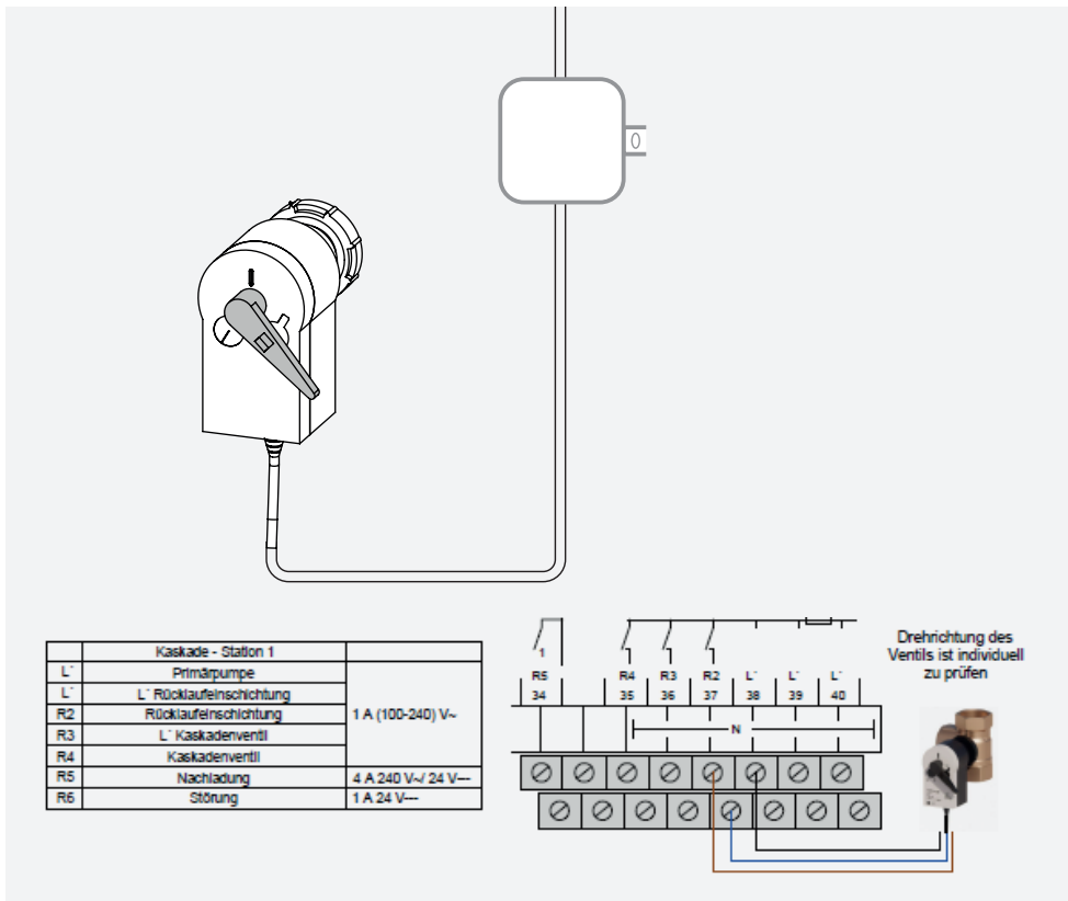
Abbildung 19 - Die geschaltete Phase des 3-Wege-Ventils wird an R2 der Kaskade Station 1 oder Einzelgerät angeschlossen Die Dauerphase des Ventils wird auf Klemme 38 angelegt.
