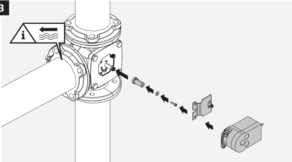
Abbildung 13 – Stecken Sie den Stellantrieb auf das Ventil.
