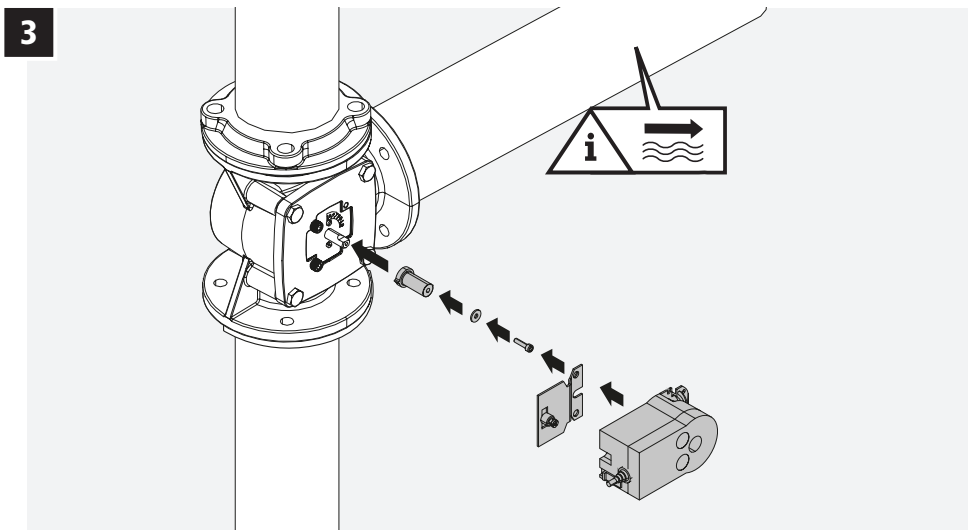
Abbildung 17 – Stecken Sie den Stellantrieb auf das Ventil.
