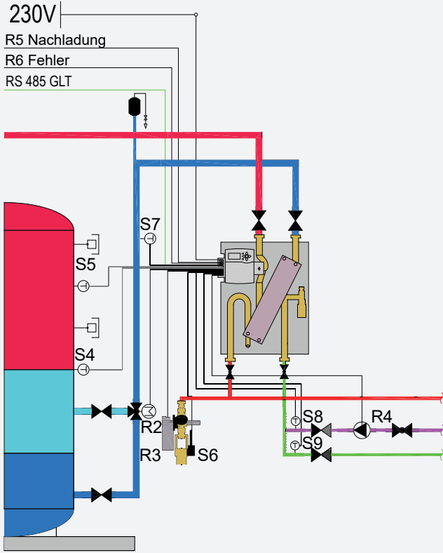
Übersicht der Aktoren und Sensoren Einzelgerät
