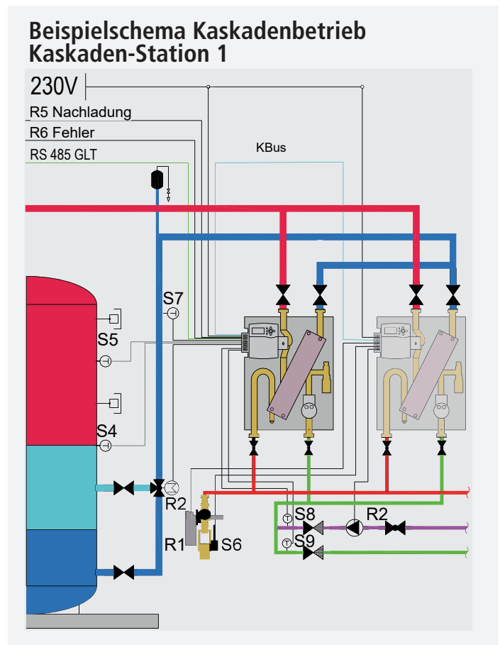
Übersicht der Aktoren und Sensoren Kaskade
