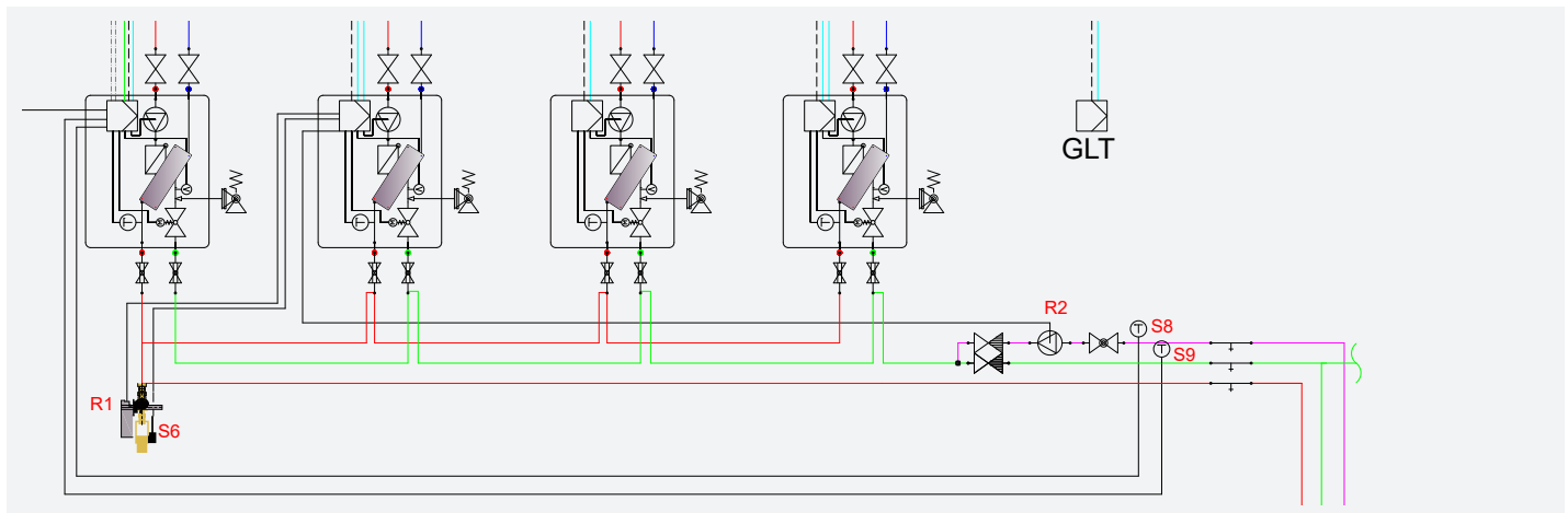
Hygienisch angeschlossene Frischwasserstationen
