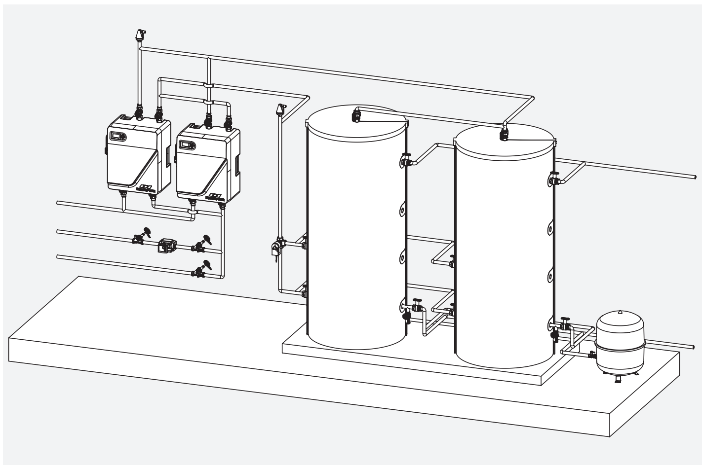
Darstellung Gesamtanlage als Kaskade
