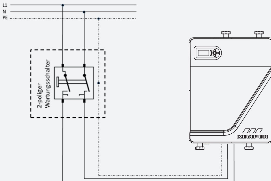
Festanschluss der Frischwasserstationen
