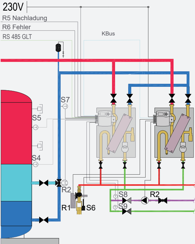
Übersicht der Aktoren und Sensoren Kaskade
