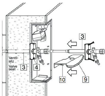
Montage Aufputz
