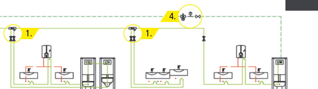
4. KHS robinetterie de mesure de la température Pt1000 Figure 628 0G
