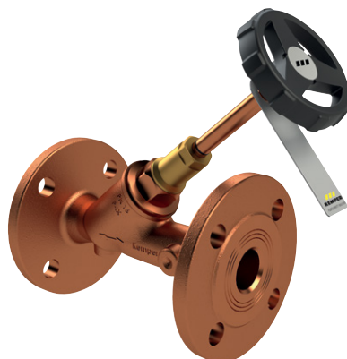
Freistrom-Absperrventil, ohne Entleerung, Flanschanschluss, Figur 135 01
