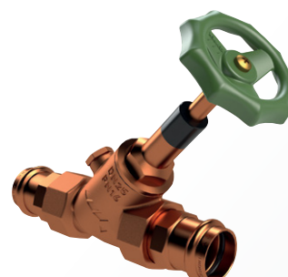
ECO Freistrom-Absperrventil, mit Entleerstopfen, mit fest inte- griertem Pressanschluss auf SANPRESS/ PROFIPRESS, Figur 171 30
