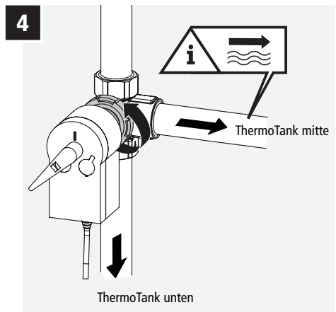
Abbildung 10 – Drehen Sie die Verriegelung um 45°, um den Stellantrieb auf dem Ventil zu fixieren.
