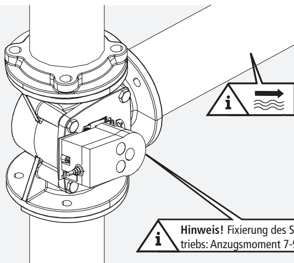
Abbildung 18 – Fixierung des Stellantriebs: Anzugsmoment 7-9 Nm.
