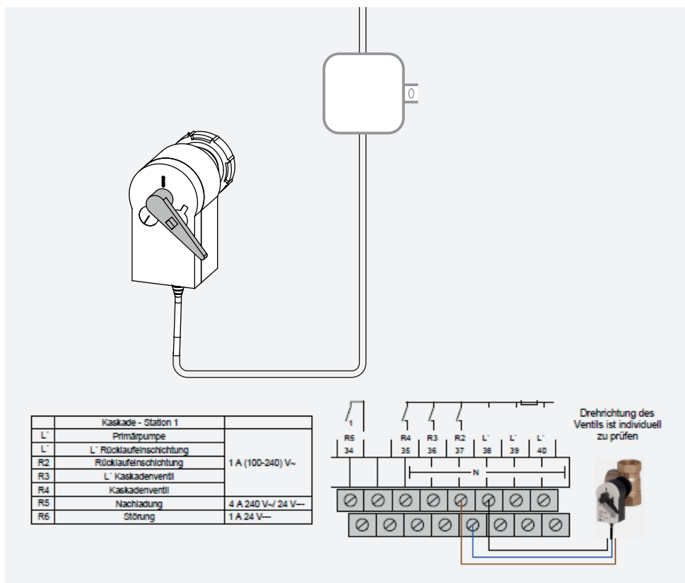
Abbildung 19 - Die geschaltete Phase des 3-Wege-Ventils wird an R2 der Kaskade Station 1 oder Einzelgerät angeschlossen. Die Dauerphase des Ventils wird auf Klemme 38 aufgelegt.
