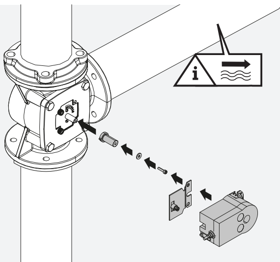
Abbildung 17 – Stecken Sie den Stellantrieb auf das Ventil.
