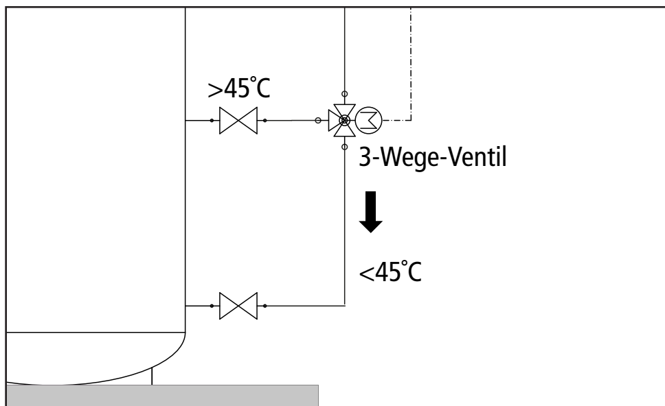
Abbildung 1 - Prinzipdarstellung 3-Wege-Umschaltventil.
