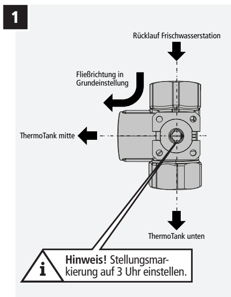
Abbildung 5 - Stellungsmarkierung.
