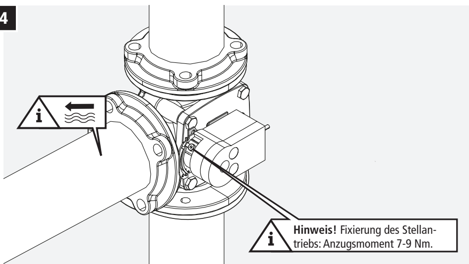
Abbildung 14 – Fixierung des Stellantriebs: Anzugsmoment 7-9 Nm.
