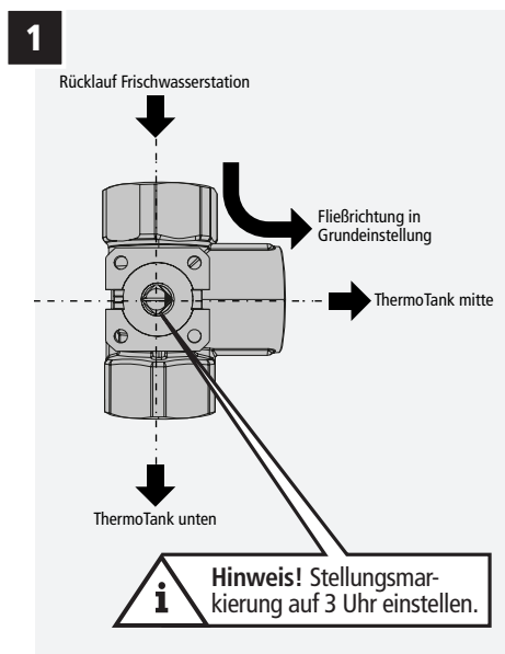
Abbildung 6 - Stellungsmarkierung.
