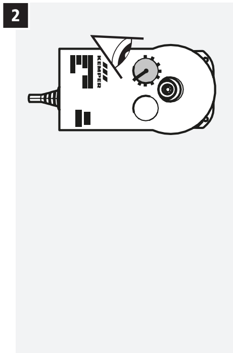
Abbildung 16 – Stellen Sie den Anschlag des Stellantriebs nach rechts (0%).
