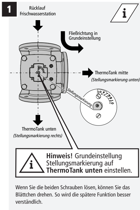
Abbildung 15 - Stellungsmarkierung.
