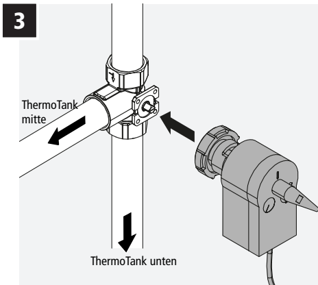
Abbildung 9 – Stecken Sie den Stellantrieb auf das Ventil.
