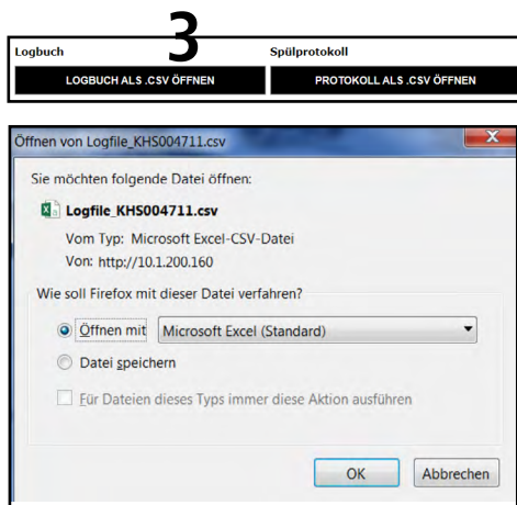
Abbildung 6.6.5: Öffnen-Dialog CSV-Logfile
