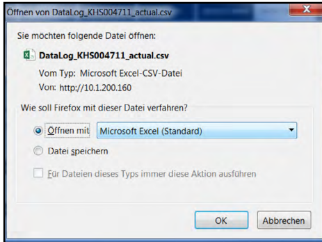
Abbildung 6.6.6: Öffnen-Dialog CSV-Datalog
