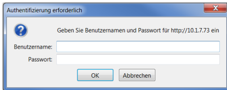
Abbildung 6.2.1: Eingabedialog Authentifizierung
